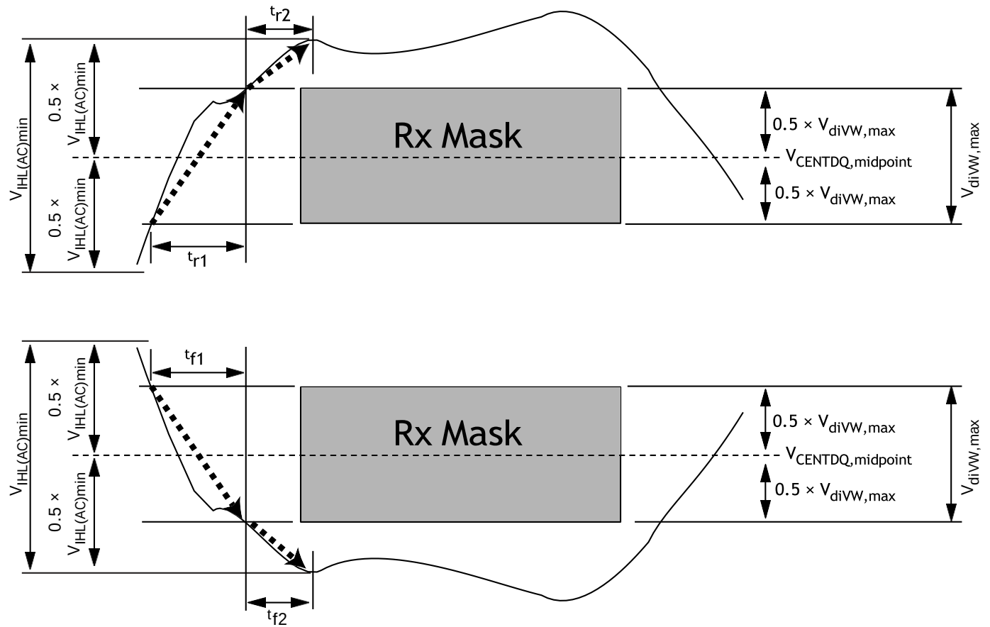
Figure 206: DQ Slew Rate Definitions
